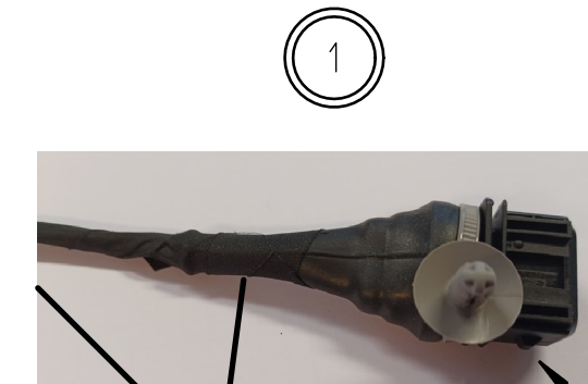
Kabellülle mit Tapeband (ca. 20mm) einwickeln Wrap the cable crommet with tape (ca. 20mm)
