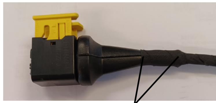
Kabellülle mit Tapeband (ca. 20mm) einwickeln Wrap the cable crommet with tape (ca. 20mm)
